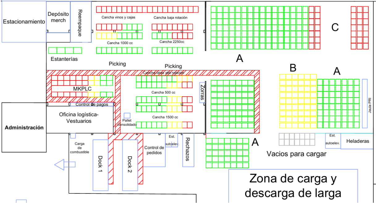
Figura 1: layout actual.
